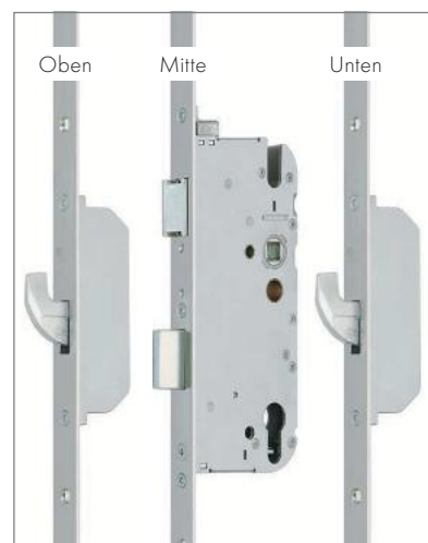
Riegelhakenschloss 3-fach
